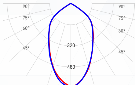
УГОЛ ИЗЛУЧЕНИЯ 90°
